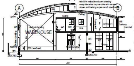
UNIT 1 SECTION A-A 1:100
